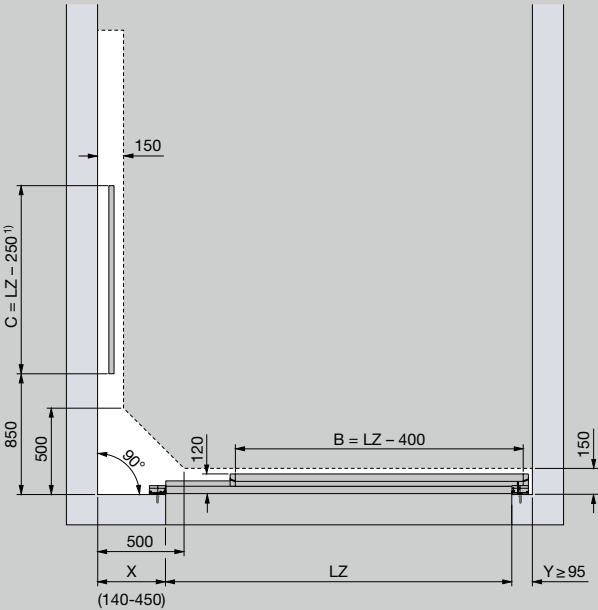
Fixation du cadre dormant haut en 1 élément
