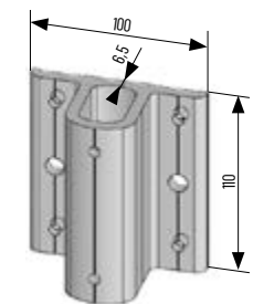
Embase Alu pose en nez de dalle L 100 x H 110 pour Givry et Montagny
