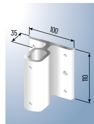
Embase Alu pose en nez de dalle L 100 x H 110 pour Chablis et Irancy
