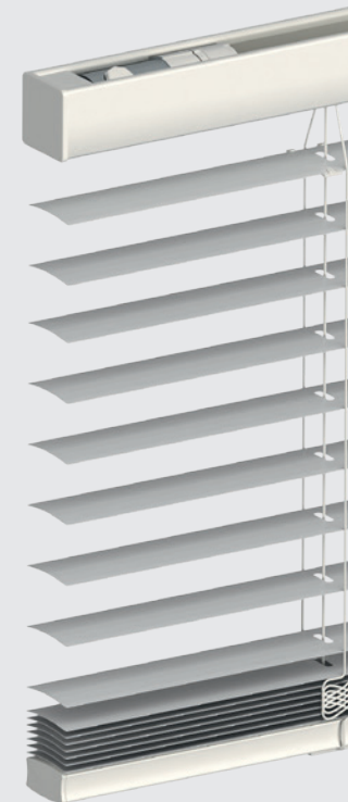
Manœuvre motorisée 24 V Somfy filaire ou radio avec choix d'émetteur mural ou portable
