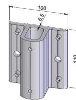
Embase Alu pose en nez de dalle (Modèles Givry et Montagny)
